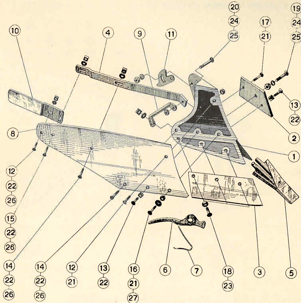
Komplett vändplogkropp, främre, 14". Detaljnummer FE 1015 » » bakre, 14". » FE 1016
