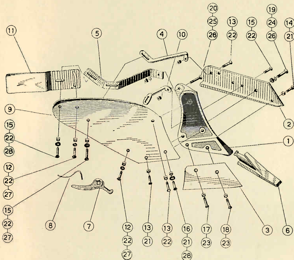
Komplett brytplogkropp, främre, 12". Detaljnummer FE 1010 » » » bakre, 12". » FE 1011
