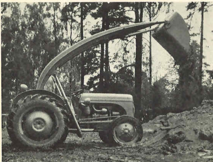
Jordskopian tippas med en hydrauliskt påverkad kolv som är placerad omedelbart bakom skopan.
