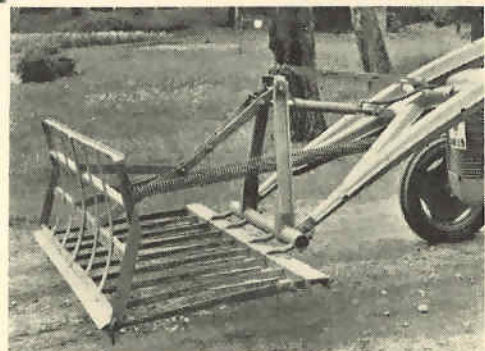
Lastapparatens försedd med katapulträfsa för bl. a. lastning och hässning av hö. På bilden är själva katapulten i sitt ytterläge.
