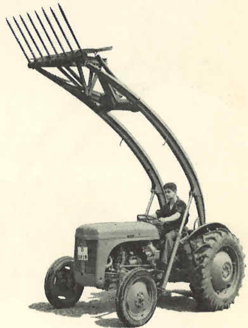
Ovanstående bild visar lastapparatens i sitt högsta läge försedd med gödselgrepp och katapult.
